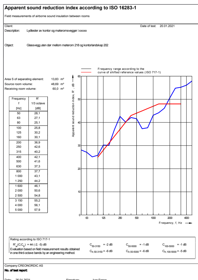
Dipp i det høyere frekvensområdet på målekurven kan tyde på lydlekkasje.
