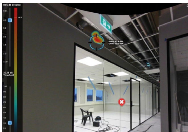
Test 3: Glassvegg i møterom med R'_w krav=34 dB. Lekkasje i skjørt. Det kan ofte være lekkasjer i forbindelse med gjennomføringer (El., Vent. og sprinkel). Se lydcurve.
